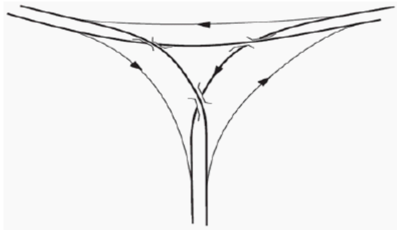
Фигура 79. Свободно планиран пътен възел тип „Триъгълник“ (7) Характеристиките на магистрален пътен възел тип „Вилица“ (фигура 80) са следните: 1. предимства: а) създава условия за равномерна скорост на транспортните потоци във всички направления; б) изисква строителството на едно мостово съоръжение;
