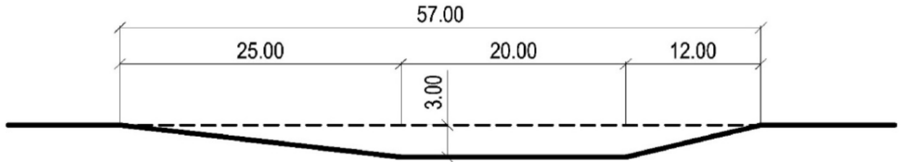
а) размери на автобусна спирка
