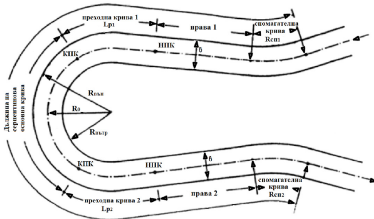
Фигура 8. Елементи на серпантината в ситуация Таблица 14 Геометрични елементи на серпантини
