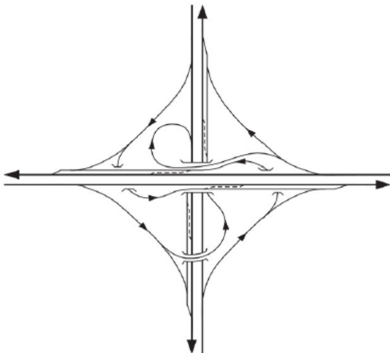
Фигура 71. Модифициран възел с рампа тип „Примка“
