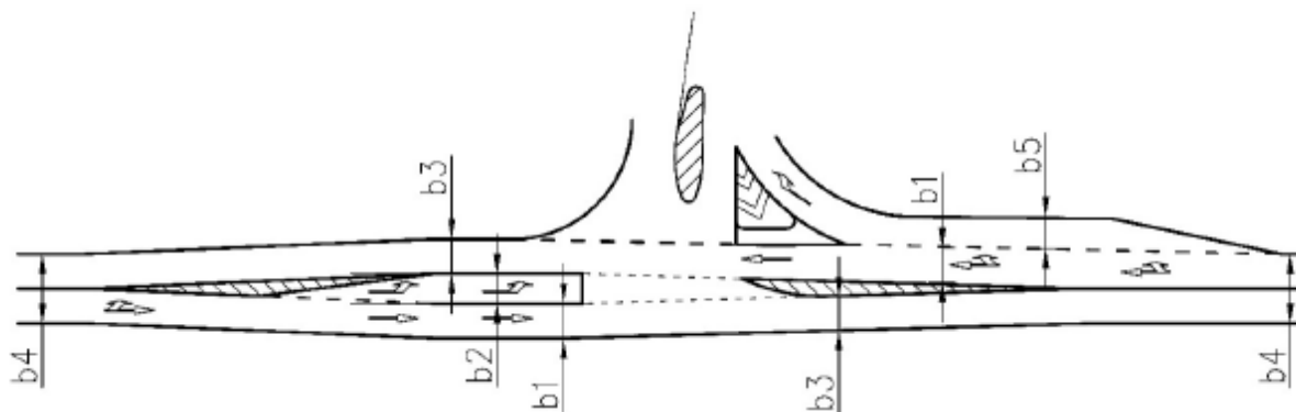
Фигура 53. Означение на широчините на допълнителните ленти при кръстовища Таблица 25
