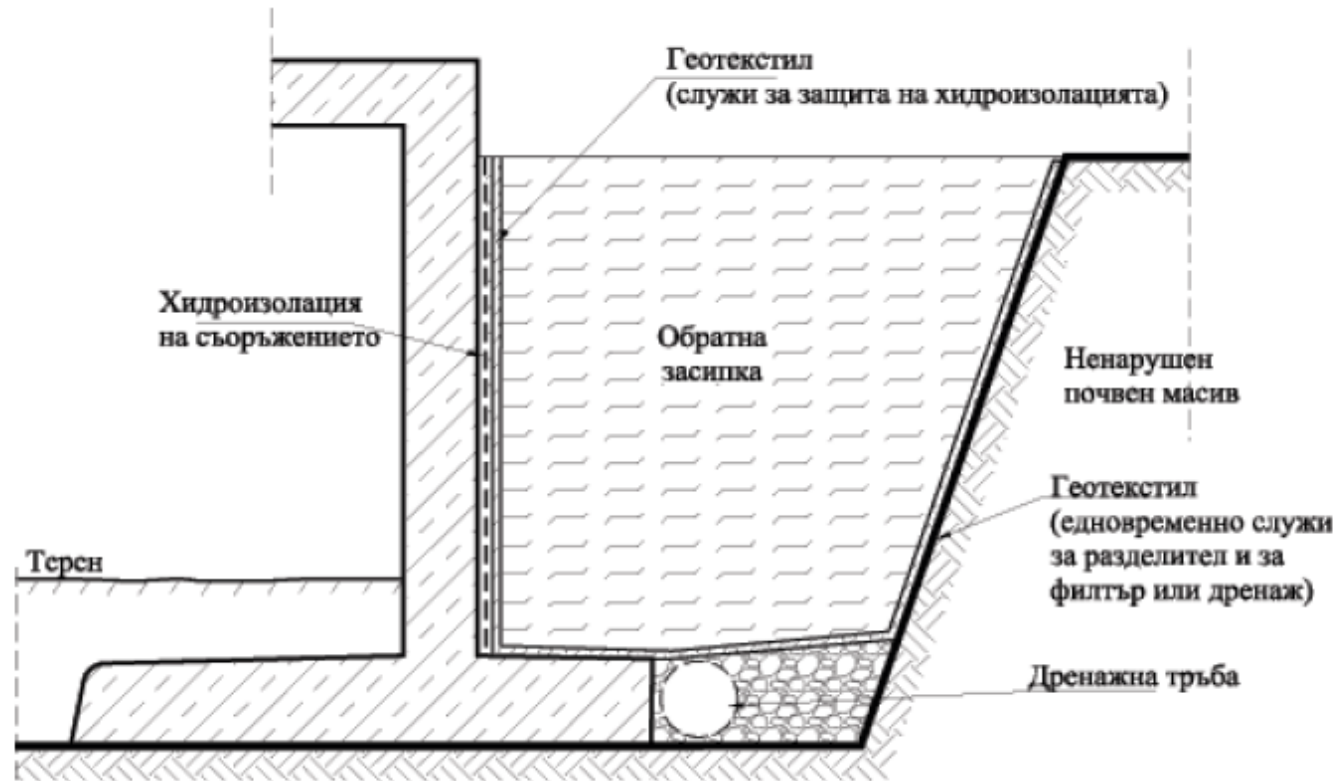
Фигура 132. Отводняване на обратната засипка: геотекстилт служи за защита на хидроизолацията на инженерното съоръжение и евентуално на дренажа (лява част); геотекстил се полага и между насипния материал и почвата 8. подпорна стена от габиони с геотекстилен филтър съгласно фигура 133;
