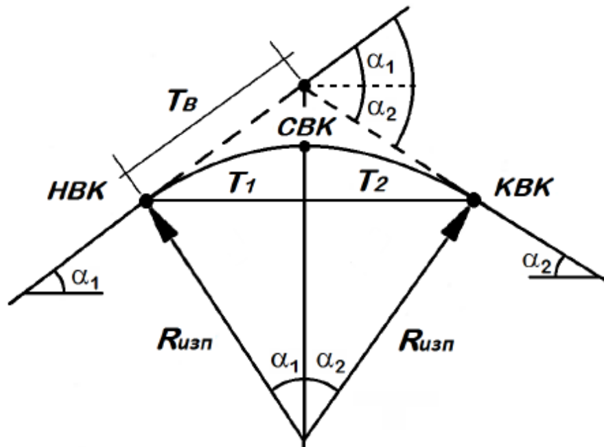
Фигура 6.2. Схема на изпъкнала вертикална крива 6.3.1. Определяне
