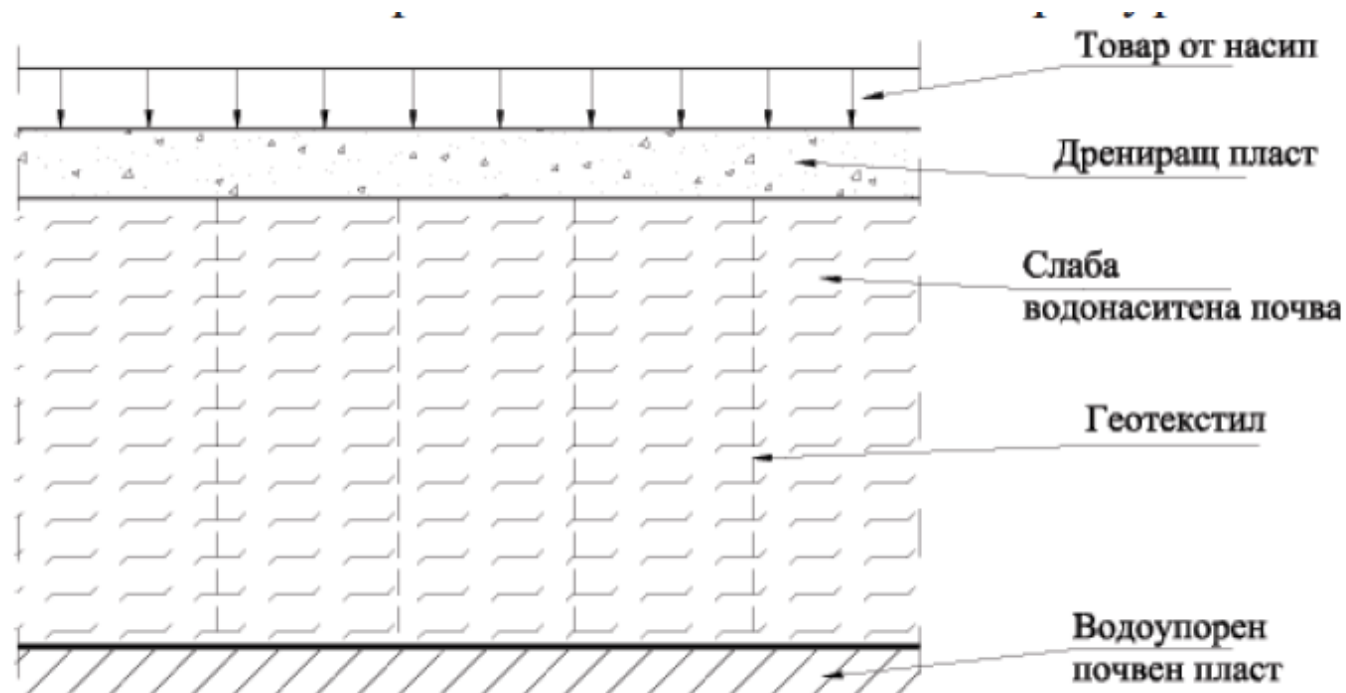
Фигура 134. Дренажна система с дренажен геокмпозит, служещ за ускоряване на консолидацията
