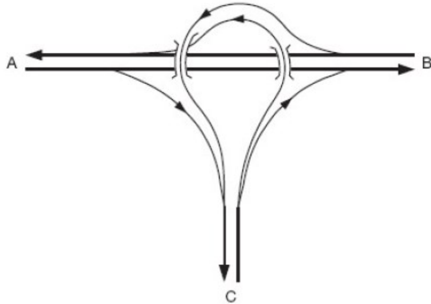
Фигура 76. Пътен възел тип „Круша“
