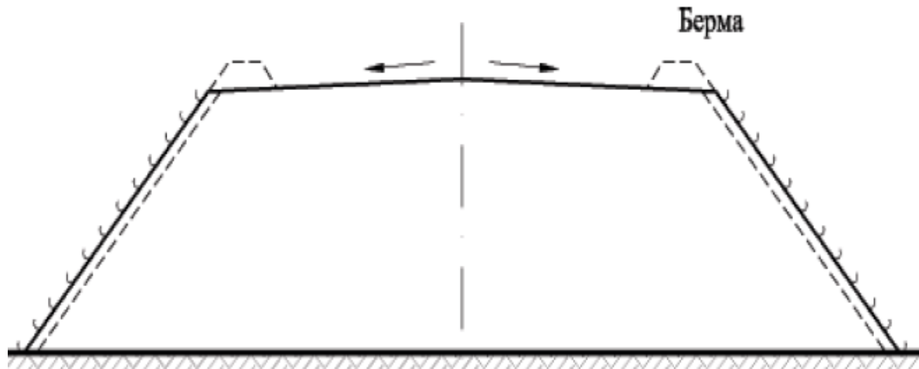
Фигура 149. Схема за затревяване и отводняване на откосите
