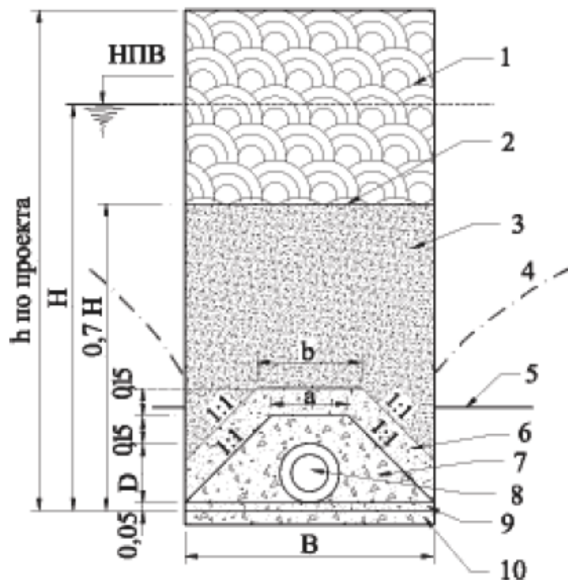
Фигура 121. Траншеен хоризонтален тръбен дренаж:
