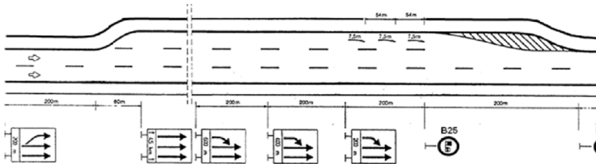
Фигура 12.1. Разположение и примерна сигнализация на допълнителна лента при нови автомагистрала с разширяване на платното от страна на средната разделителна ивица
