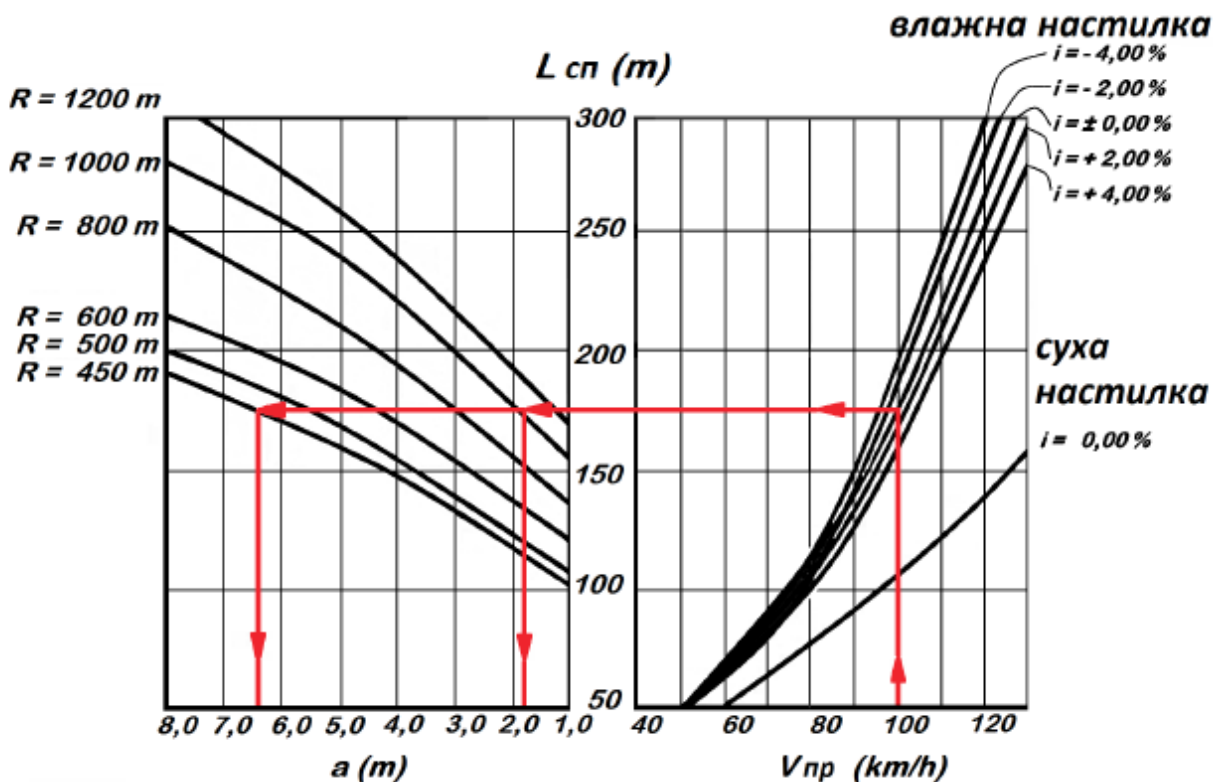
Фигура 10.3. Номограма за отчитане на L_{сн} и a^H за проверка на страничното разстояние за видимост
