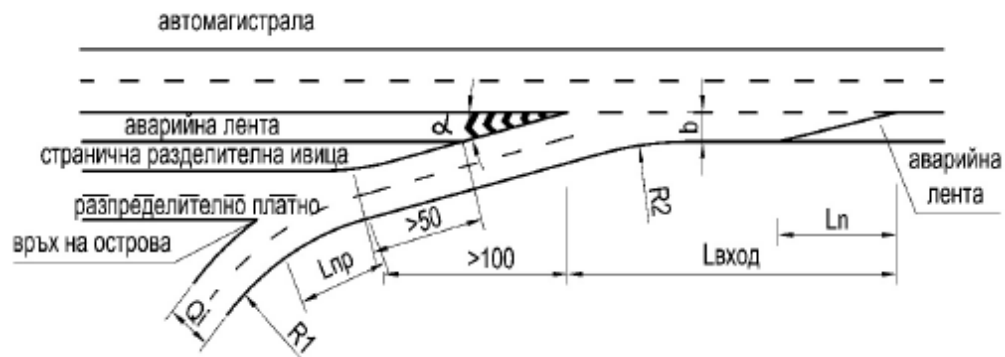
Фигура 95. Вход при разпределително платно
