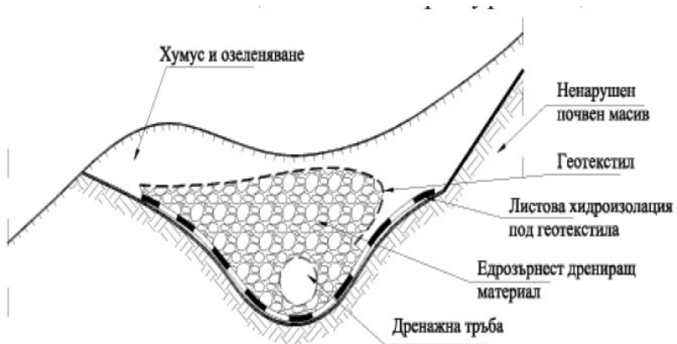
Фигура 130. Предпазен окоп, комбиниран с подокOPEN дренаж, изпълнен с геотекстил б. площен дренаж под голям наклон, комбиниран с отвеждане на водата в подокOPEN дренаж с геотекстил, съгласно фигура 131;
