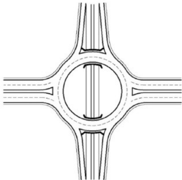
Фигура 62. Кръгово кръстовище с две съоръжения
