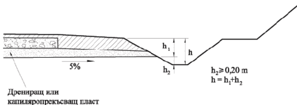
Фигура 108. Определяне на дълбочината на пътния окоп
