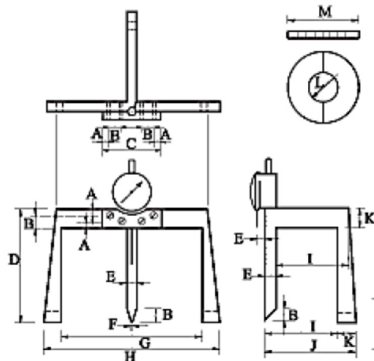
Триножен статив за определяне на набъването
