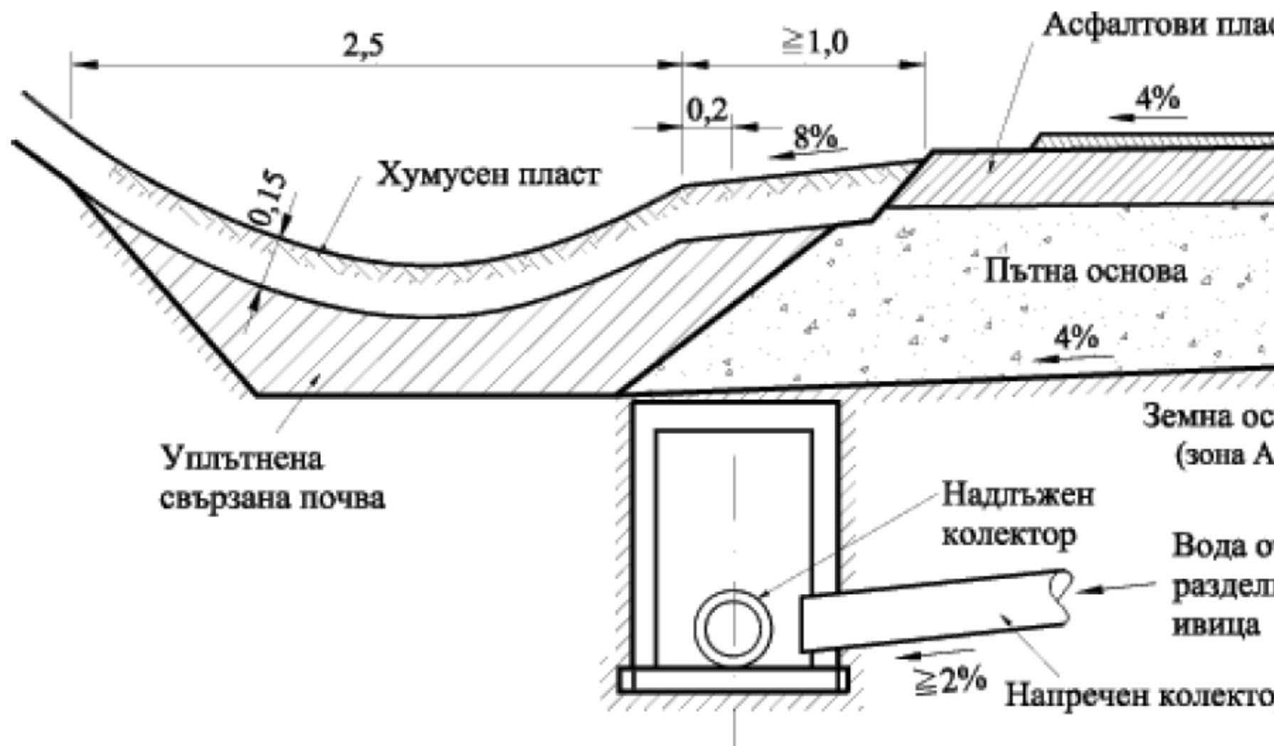
Фигура 137. Съоръжения за странично отвеждане на водите от разделителната ивица в изкоп (2) Случайно инфилтриралата през хумусния пласт на разделителната ивица вода се отвежда в надлъжния дренаж чрез напречен наклон (6,00 %) на земната основа.
