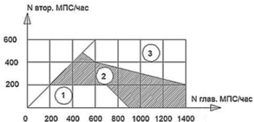
Фигура 41. Диаграма за избор на типа пътен възел и кръстовище
