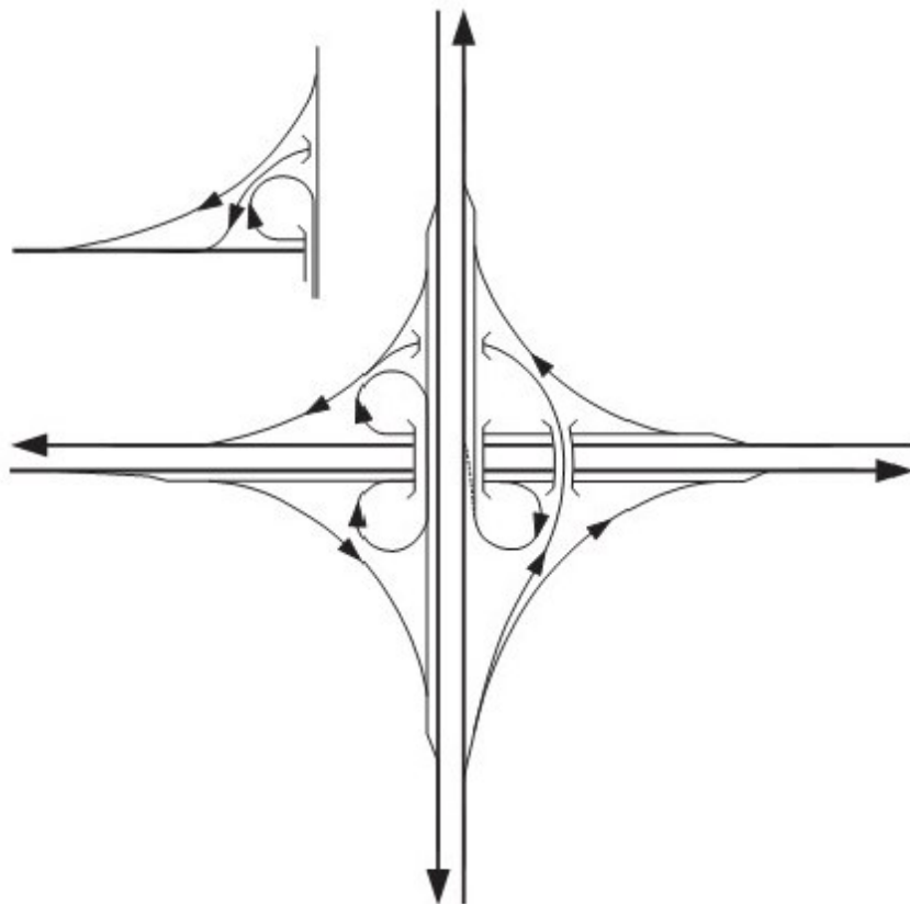
Фигура 67. Модифицирана „Детелина“ с полудиректна връзка
