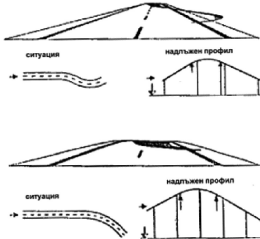
Фигура 21. Начало на хоризонтална крива във вертикална крива
