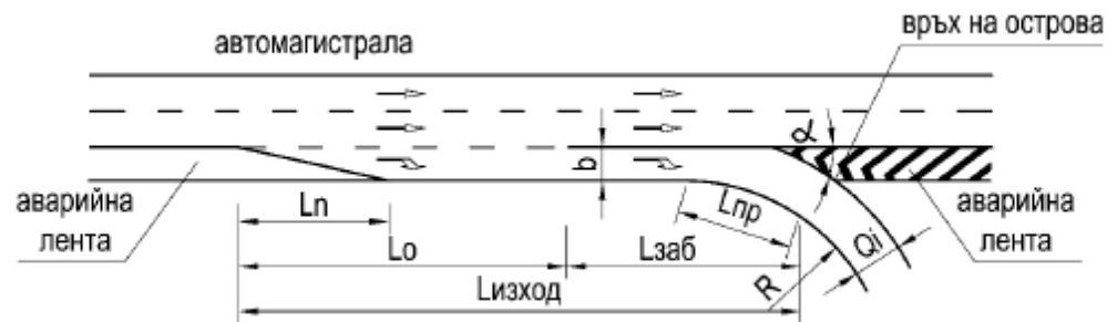
Фигура 92. Изход при директни и индиректни връзки
