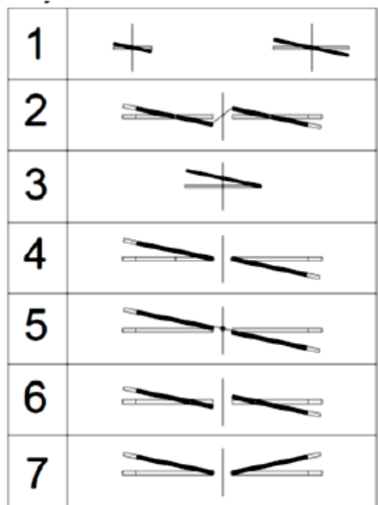
Фигура 6. Схеми на въртене на платното за движение в криви Забележка.
