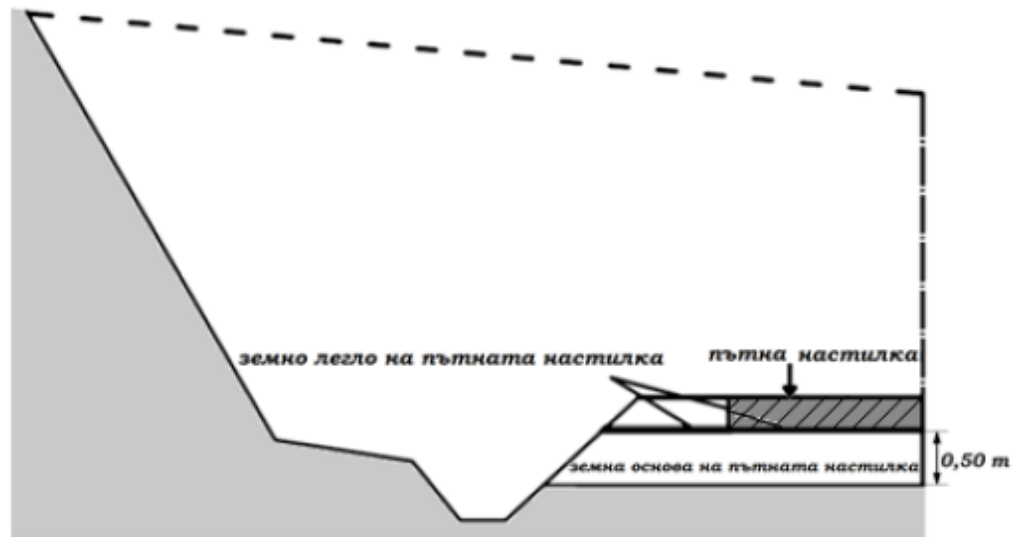
Фигура 98. Зони при насип и изкоп
