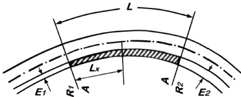
Фигура 7.3. Уширение при яйцевидна клотоида: където:
