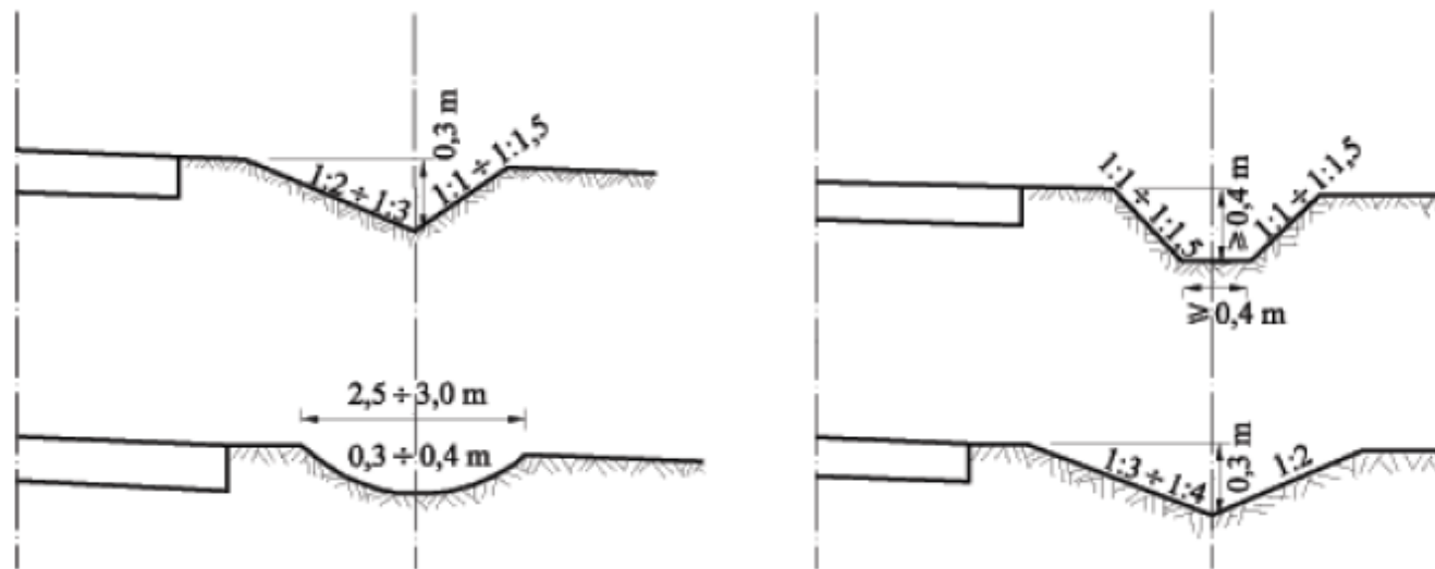
Фигура 107. Напречни сечения на пътни окопи
