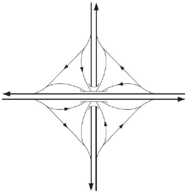
Фигура 72. Възел тип „Малтийски кръст“
