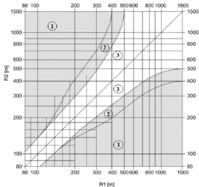
Фигура 1. Гранични съотношения между радиусите на съседни криви Забележка.
