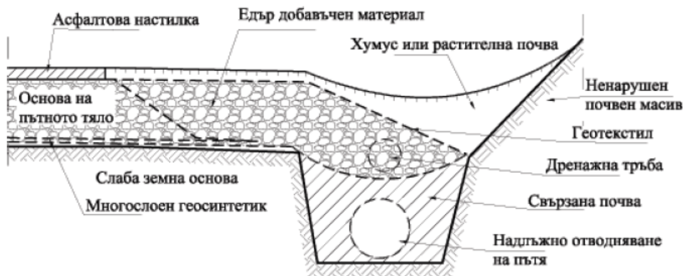
Фигура 127. Подокопен дренаж при надлъжно отводняване на пътя 3. площен дренаж, свързан с надлъжното отводняване, съгласно фигура 128;
