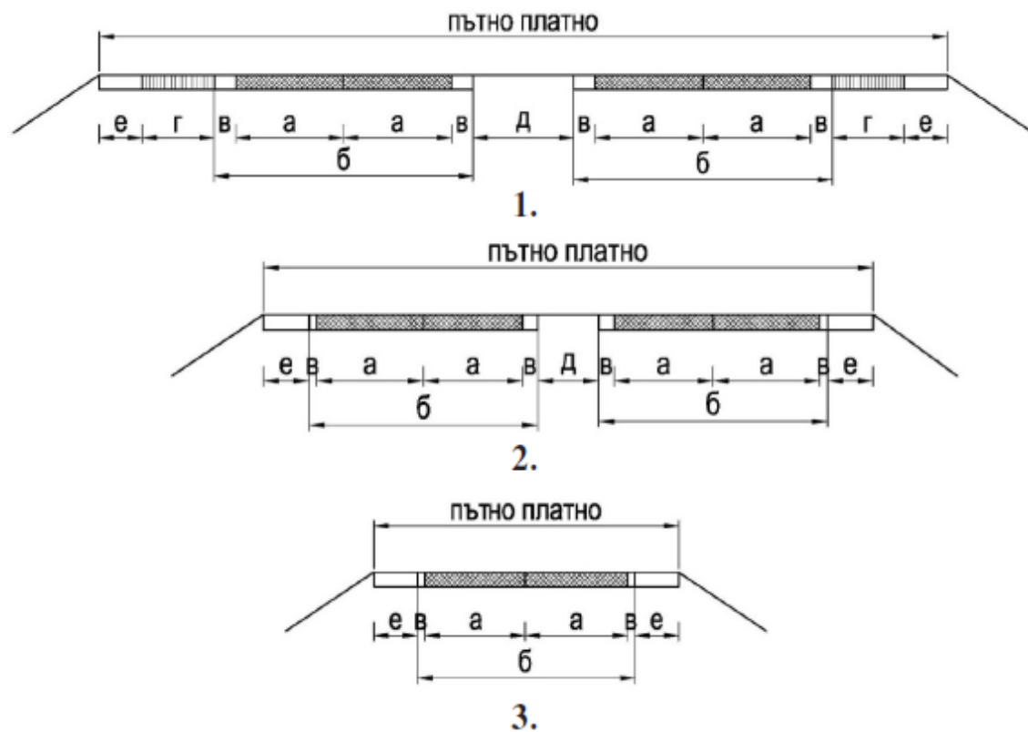
Фигура 30. Елементи на пътното платно
