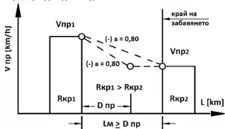
Фигура 1.1. Схема за намаляване на скоростта
