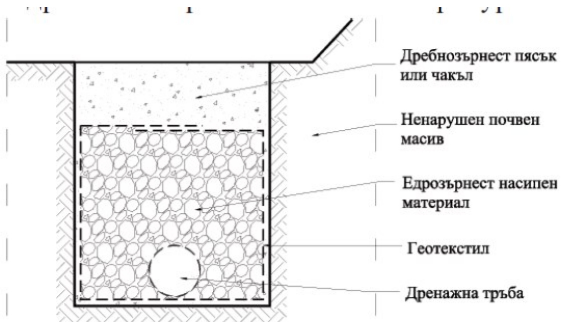
Фигура 126. Дренажна траншея
