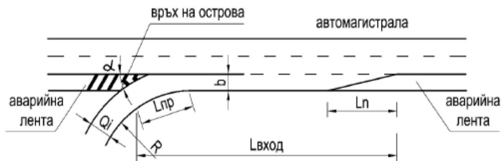
Фигура 94. Вход при директна и индиректна връзка
