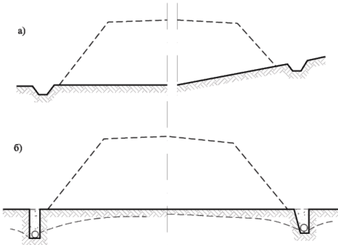
Фигура 144. Схема на отводняване на насипите преди започване на изпълнението им
