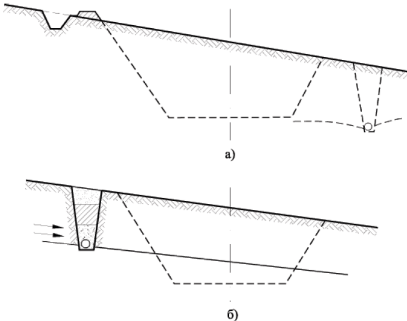
Фигура 138. Предпазни окопи и дренажи
