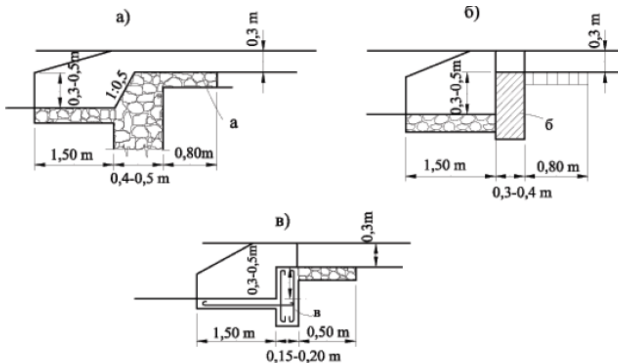
Фигура 112. Прагове в окопи ( i > 5\% ):
