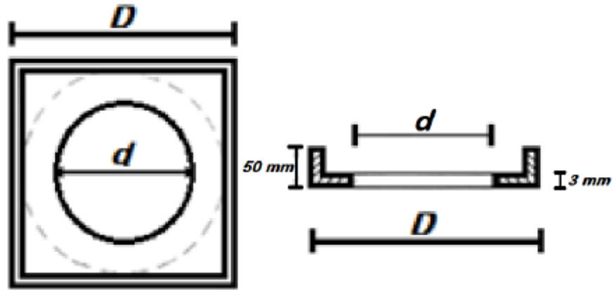
Фигура 18.1. Стоманена тава
