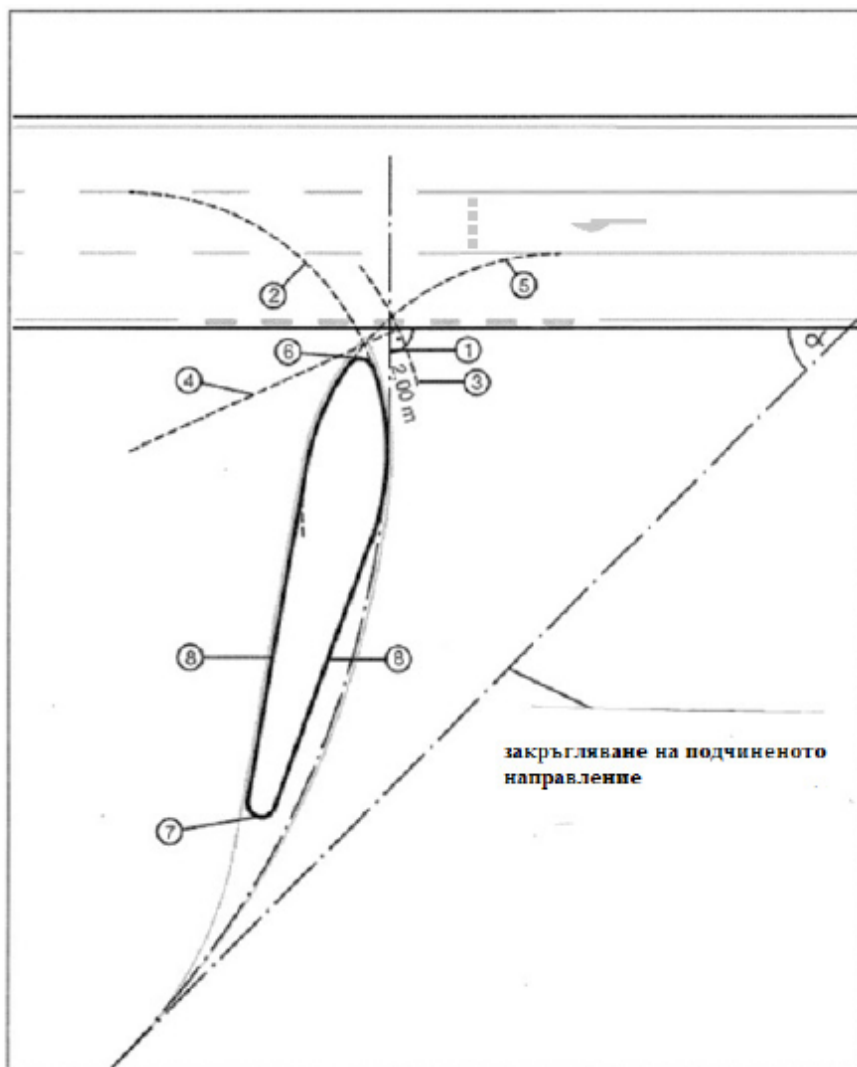
Фигура 13.5. Конструирание на голяма капка при ъгъл на пресичане \alpha < 80 \text{ gon}
