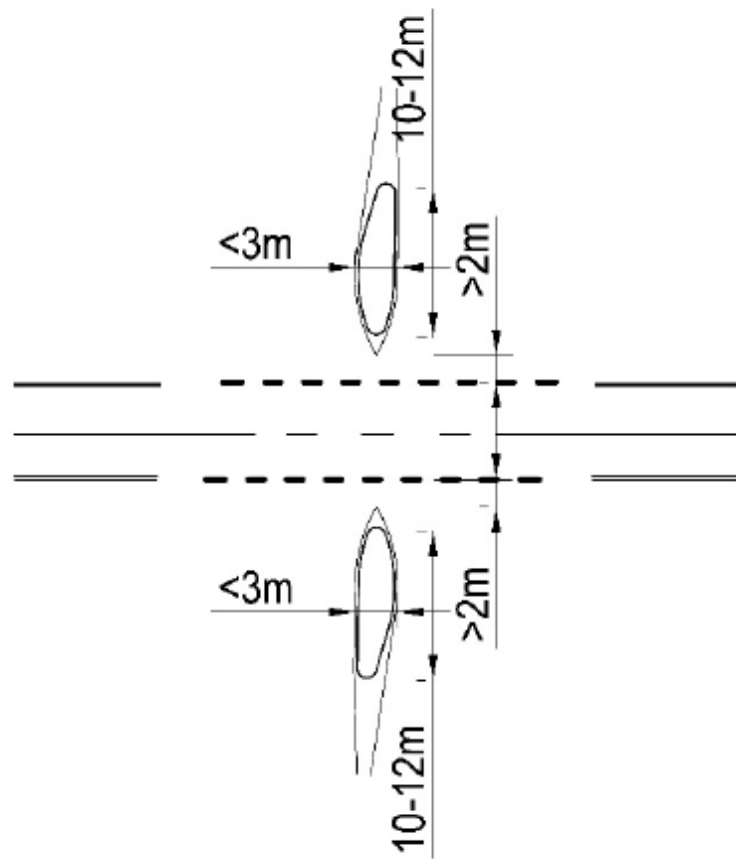
Фигура 58. Капковиден остров за кръстовища I тип
