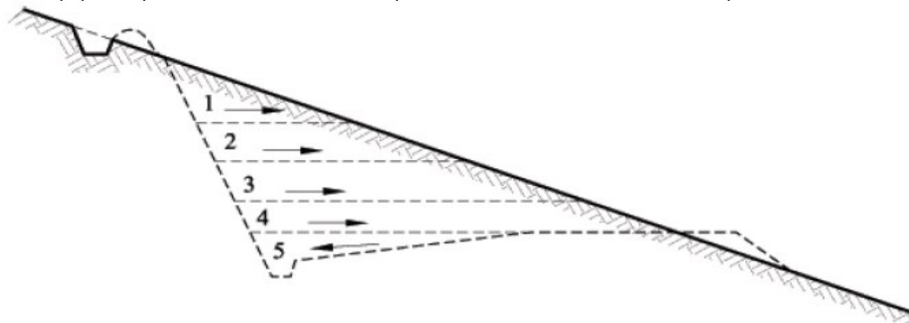
Фигура 140. Отводняване на скатен изкоп
