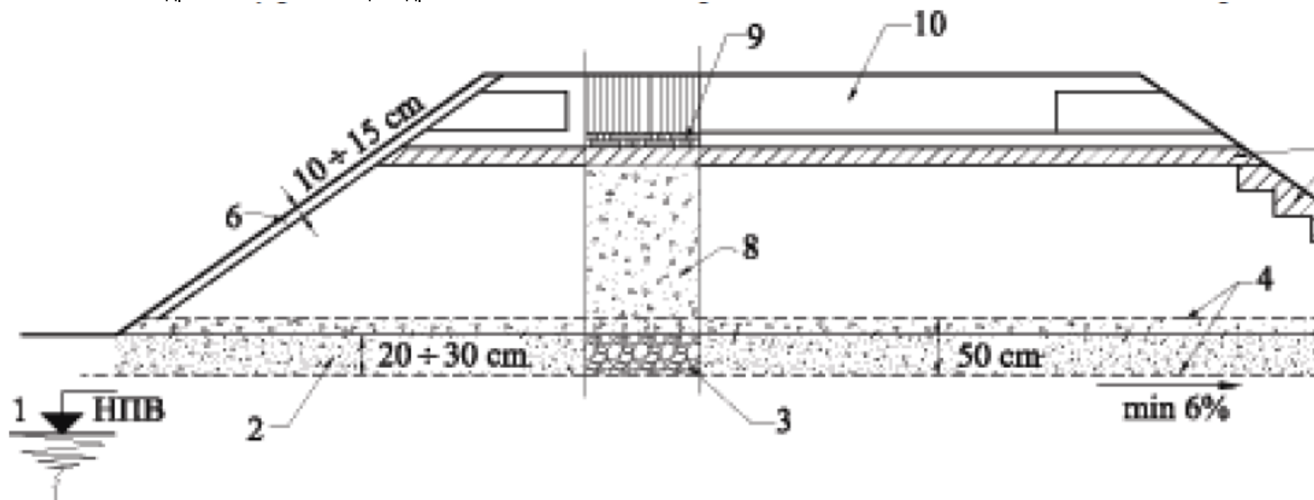
Фигура 119. Система от дренажна възглавница и дренажни пилоти
