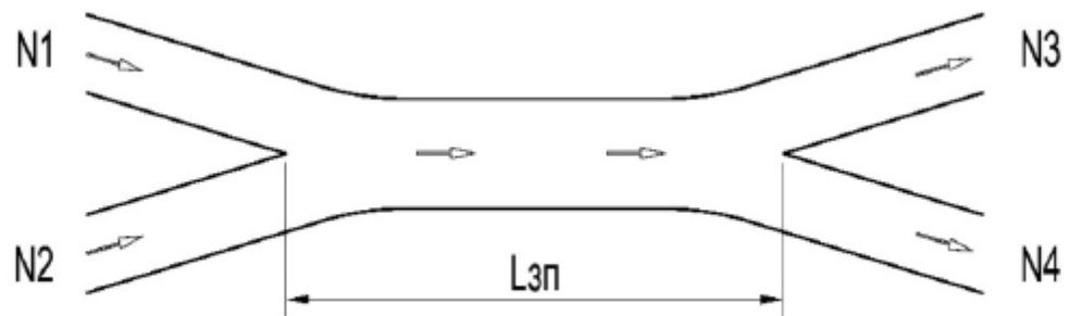
Фигура 96. Зона на преплитане
