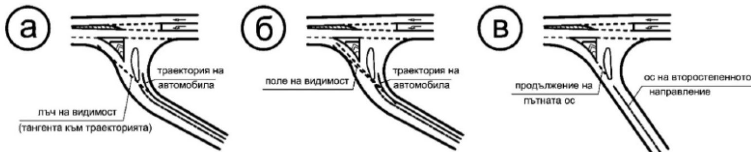
Фигура 60. Удължение на капковидния остров
