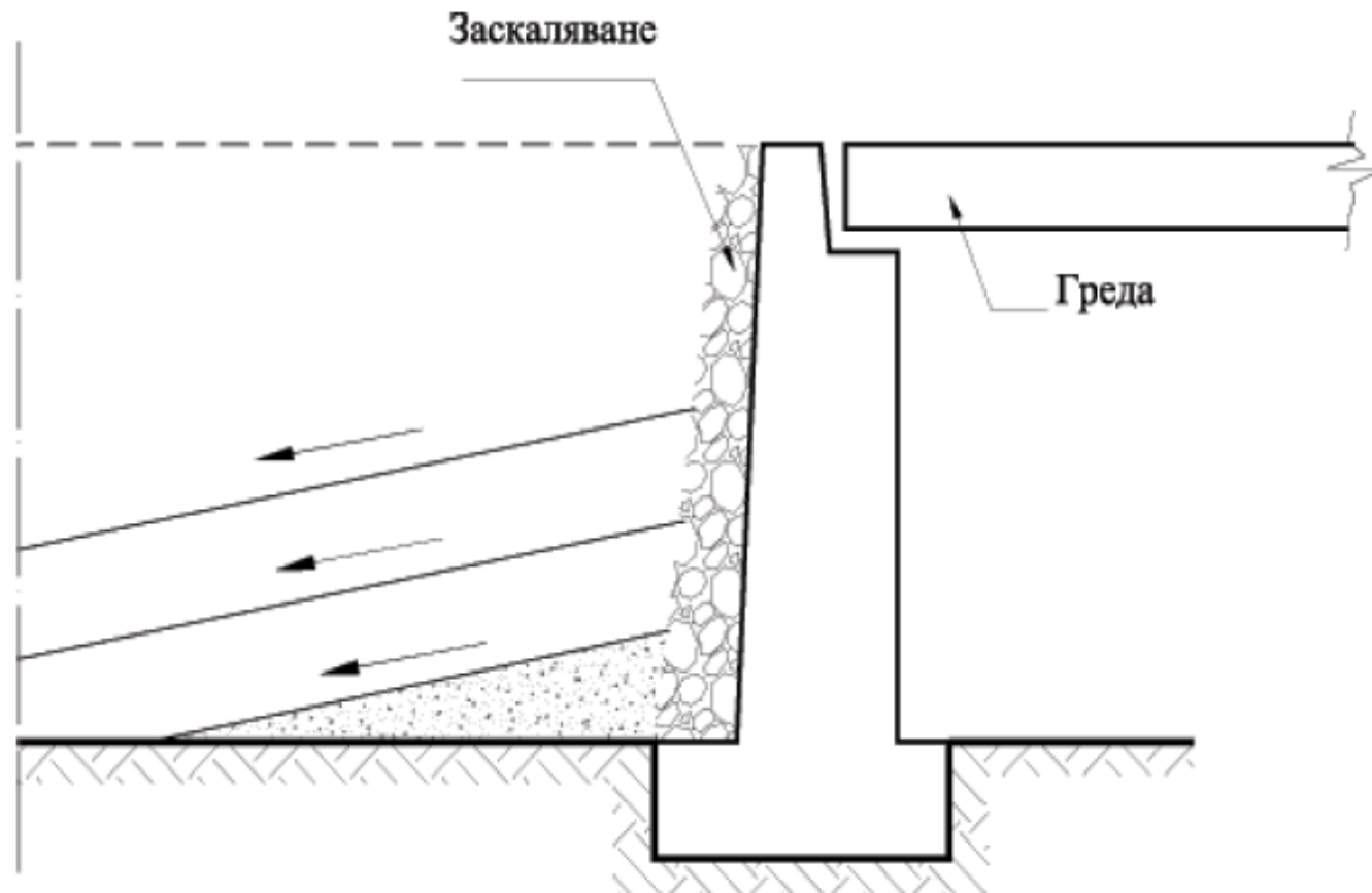
Фигура 148. Схема за изпълнение на пластове зад устой на мост
