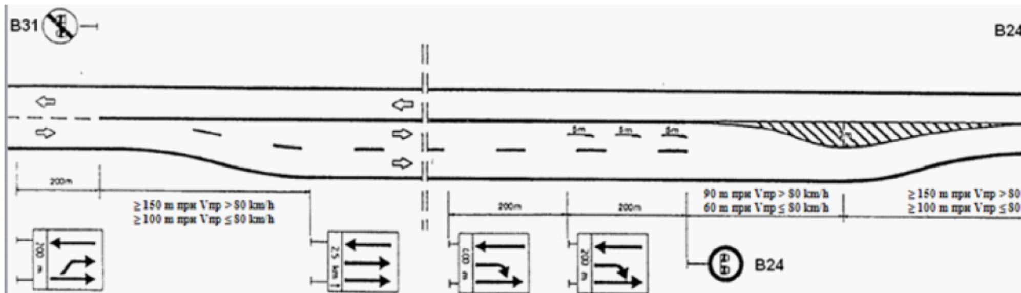
Фигура 12.4. Разположение и примерна сигнализация на допълнителна лента при двулентови пътища
