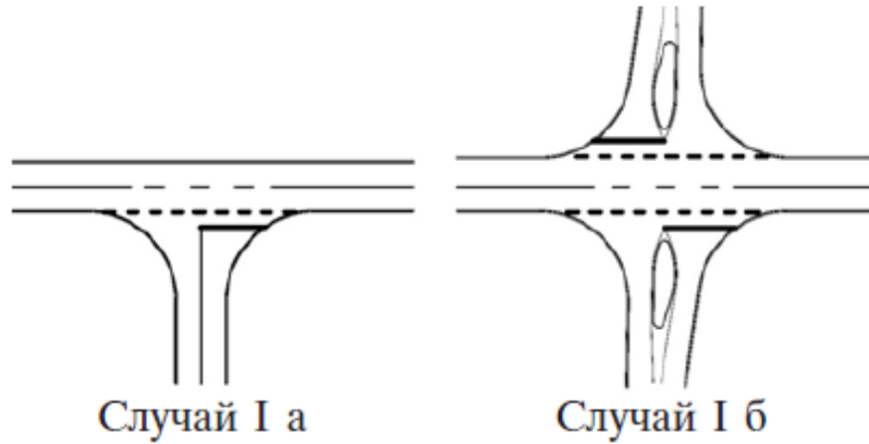
Фигура 47. Кръстовица от I тип
