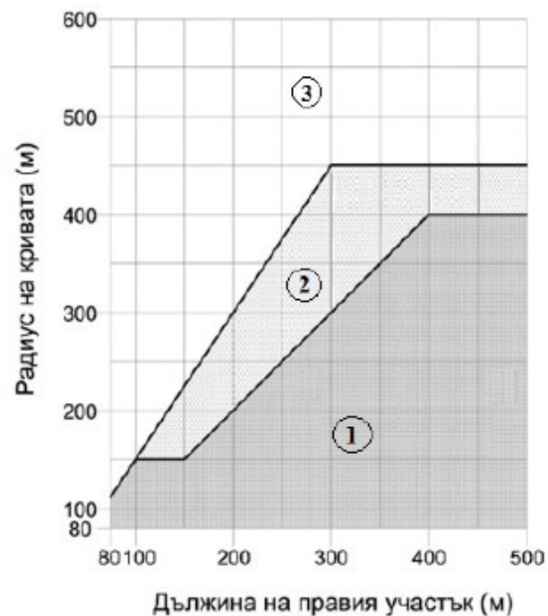
Фигура 2. Радиуси на хоризонтални кръгови криви след права Забележка.
