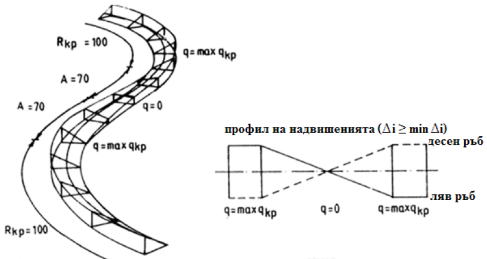
Фигура 8.1. Къса отсечка на преоформяне
