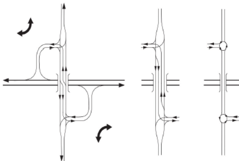
Фигура 83. Диагонална „Полудетелина“ с излизане след мостовото съоръжение (5) Характеристиките на симетрична „Полудетелина“ (фигура 84) са следните:
