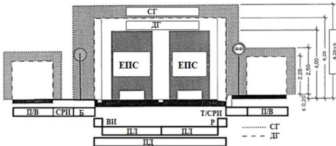
Фигура 31. Пътни габарити
