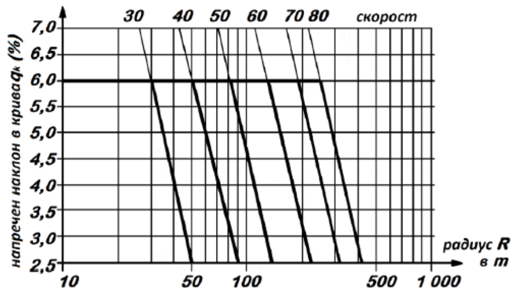
Фигура 91. Напречни наклони при пътни връзки
