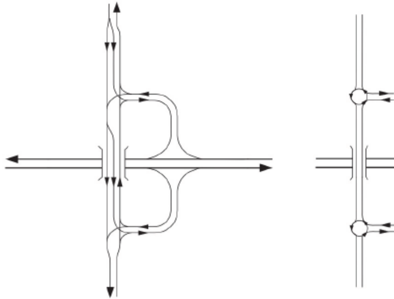
Фигура 84. Симетрична „Полудетелина“
