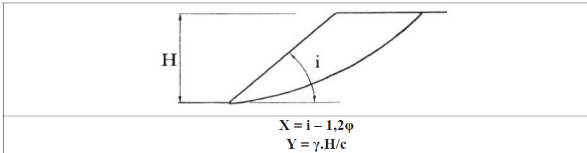
Фигура 102. Дрениран откос без опънна пукнатина
