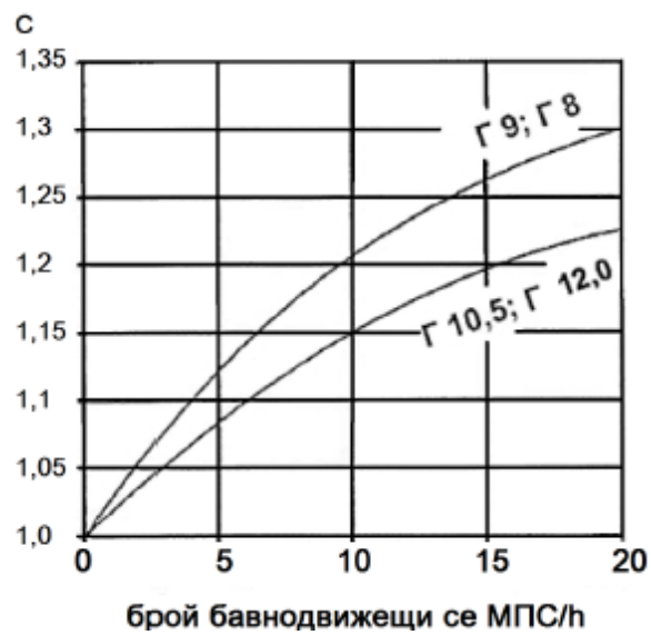
Фигура 11.2. Коефициент на влияние на бавнодвижещи се МПС (БМПС)
