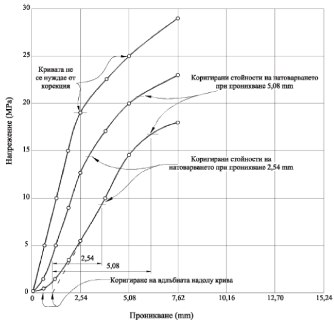
Фигура 17.2. Корекция на кривата „напрежение - проникване“
