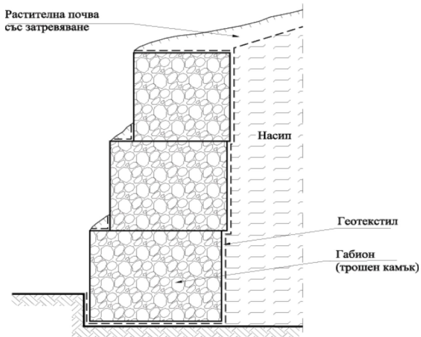
Фигура 133. Стена от габиони с геотекстилен филтър 9. дренажна система с геотекстил за понижаване на порния натиск съгласно фигура 134.
