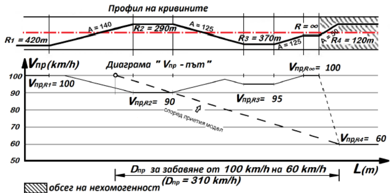
Фигура 1.5. Примерна диаграма „скорост - път“
