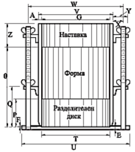
Перфорирана плоча с регулируемо стебло
