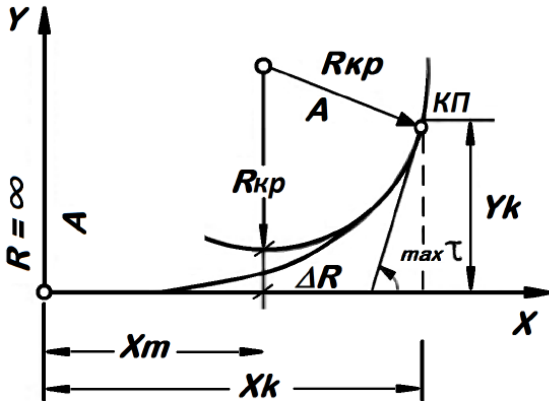
Фигура 4.2. Геометрия на клотоидата
