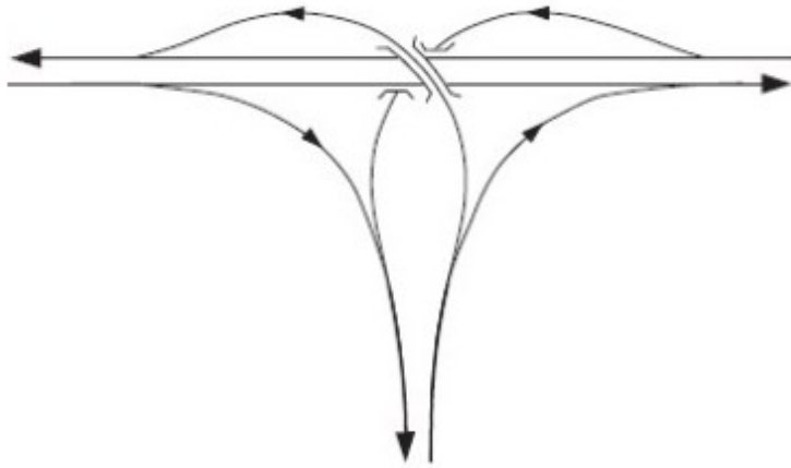
Фигура 77. Пътен възел тип „Триъгълник“ на три нива с разделени пътни връзки
