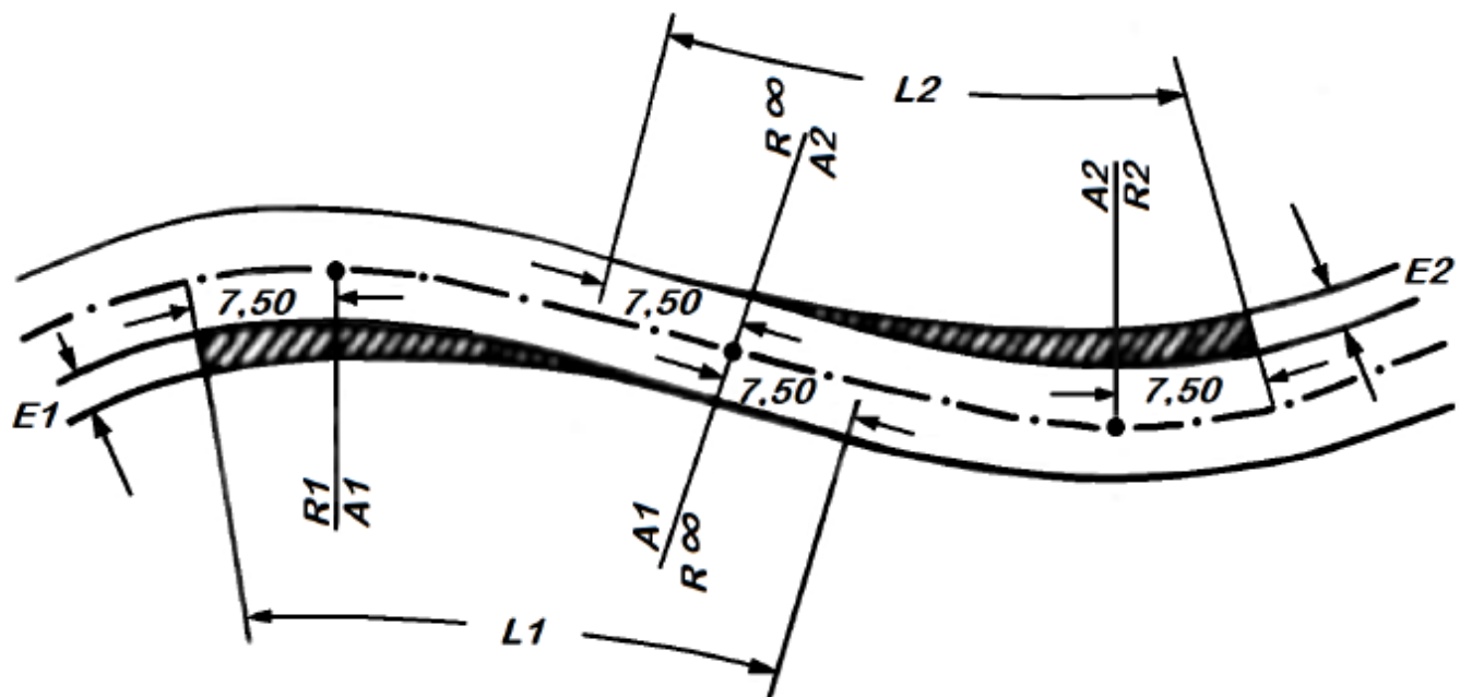
Фигура 7.4. Уширение на настилката при инфлексна клотоида
