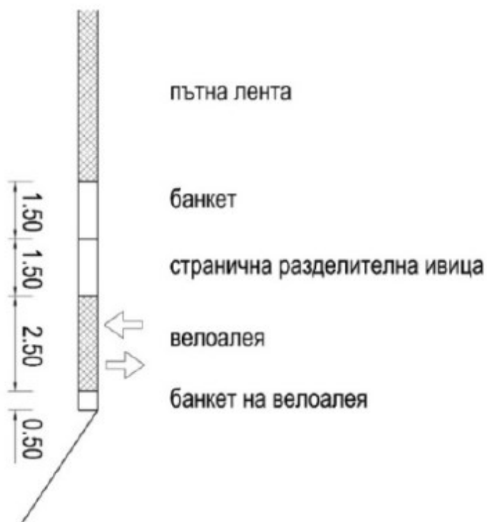
Фигура 37. Общи пешеходни алеи и алеи за велосипедисти със странична разделителна ивица при Г 10,5; Г 9; Г 8 и Г 6 Таблица 21
