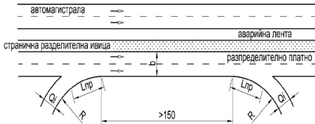
Фигура 97. Зона на преплитане към допълнителна лента, отделена от автомагистрала със странична разделителна ивица
