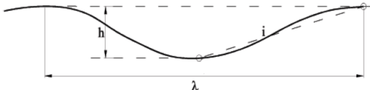
Фигура 106. Елементи на надлъжно огъната пътна конструкция вследствие консолидиране на насипа Таблица 44
