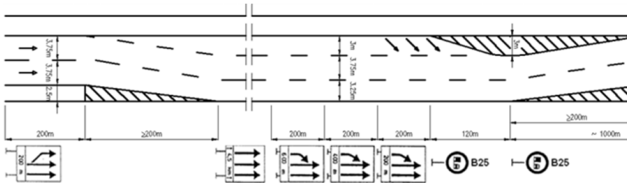
Фигура 12.3. Разположение и примерна сигнализация на допълнителна лента при съществуващи автомагистралаи
