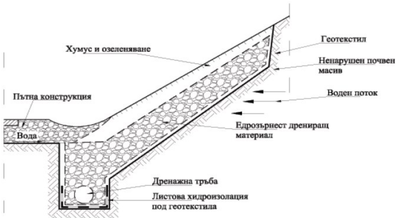
Фигура 128. Площен дренаж, свързан с надлъжното отводняване
