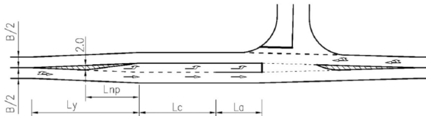
Фигура 51. Допълнителна лента ЛД
