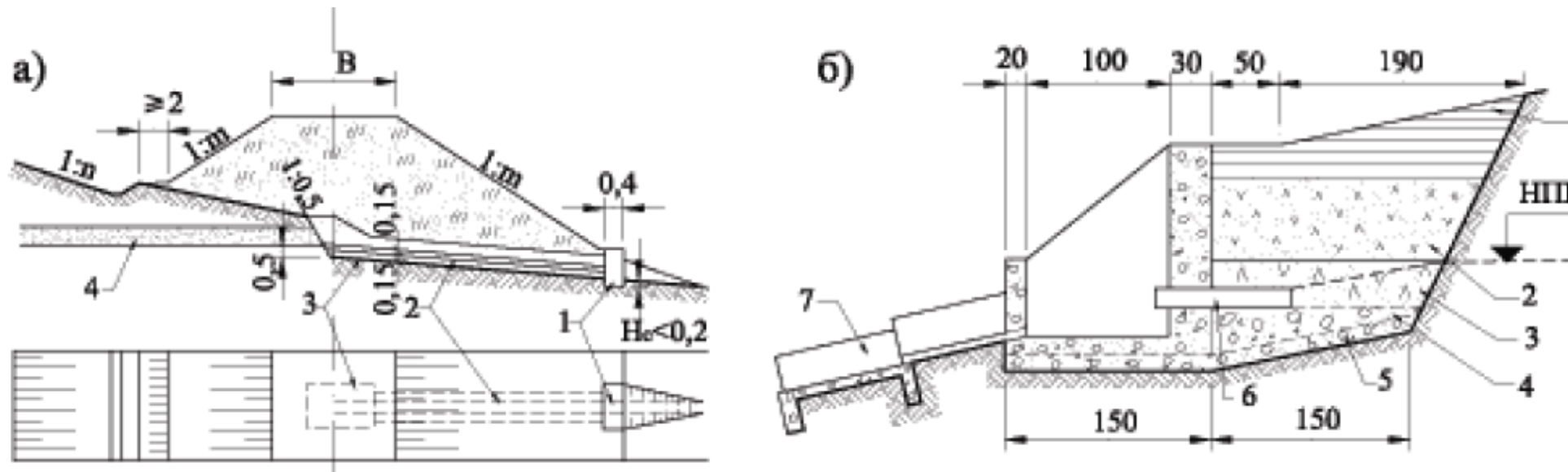
Фигура 125. Каптажи:
