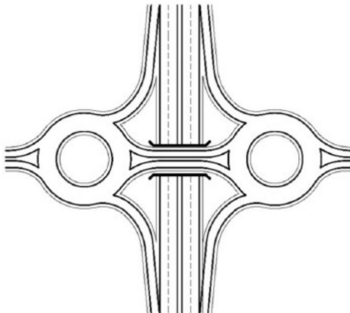
Фигура 63. Кръгово кръстовище с едно съоръжение
