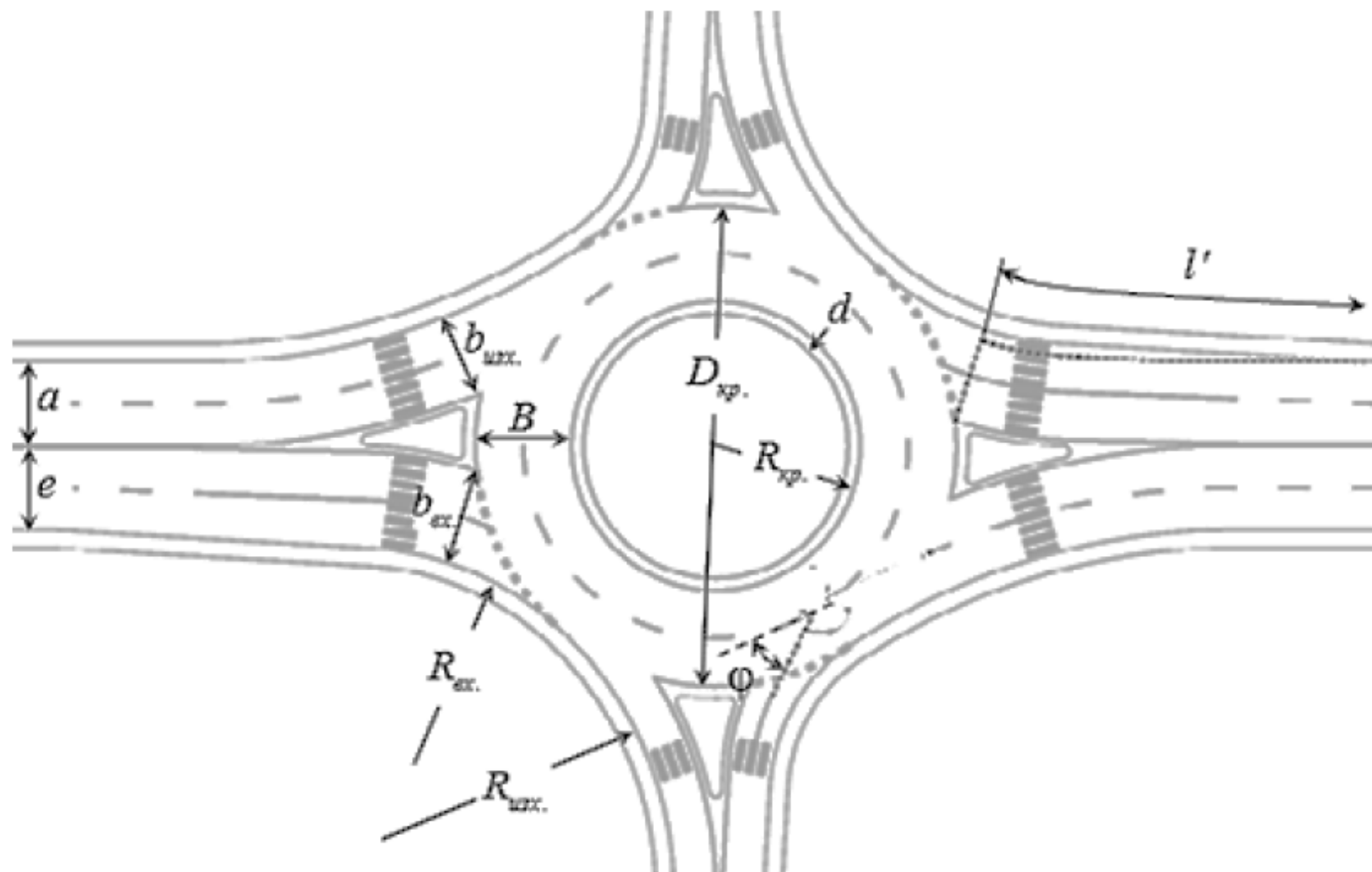
Фигура 64. Геометрични елементи на кръгово кръстовище
