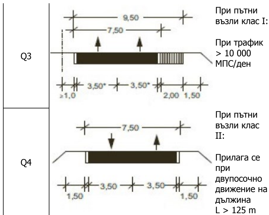
Фигура 90. Типове габарити на пътни връзки
