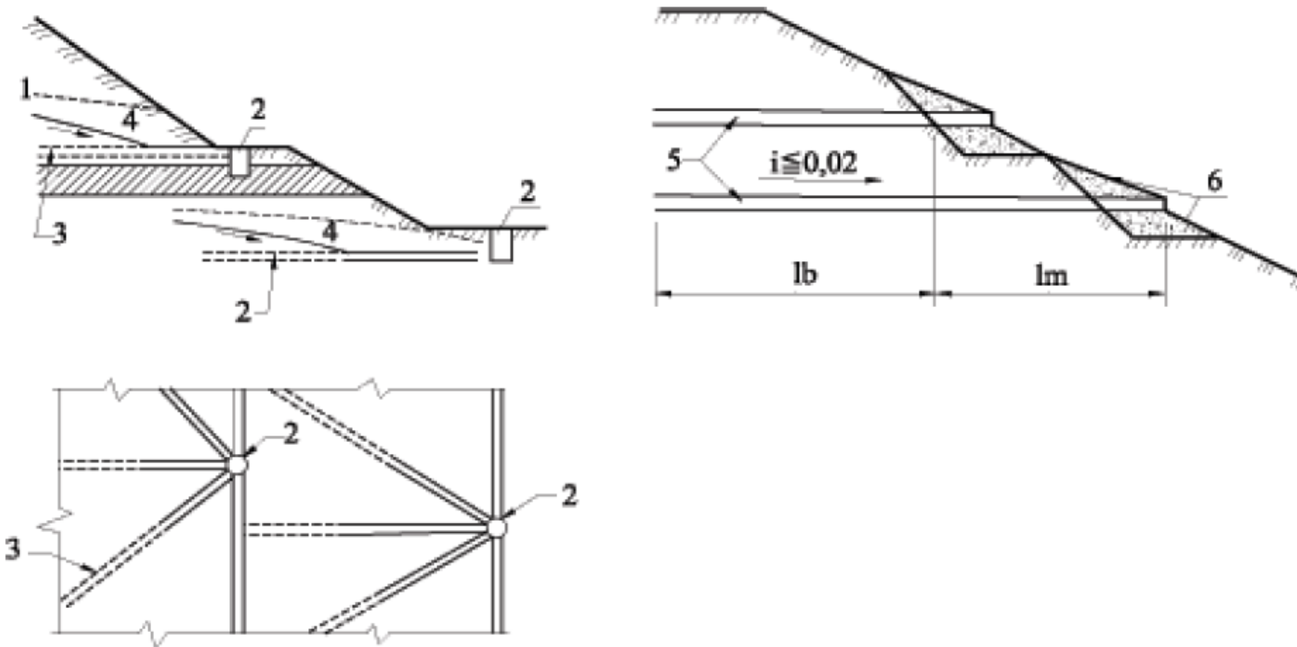
Фигура 118. Горизонтални дренажи:
