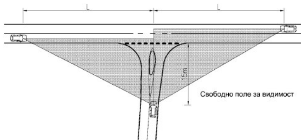
Фигура 42.б. Поле за видимост при приближаване
