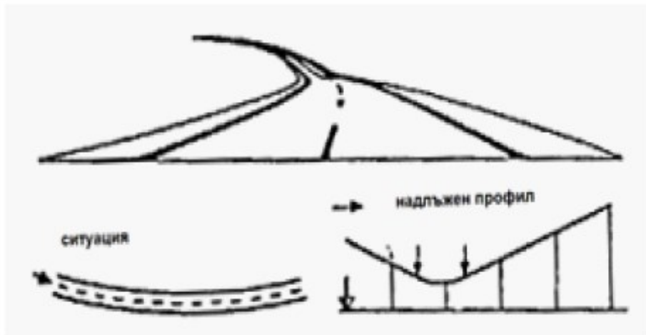
Фигура 17. Оптическо сплескване
