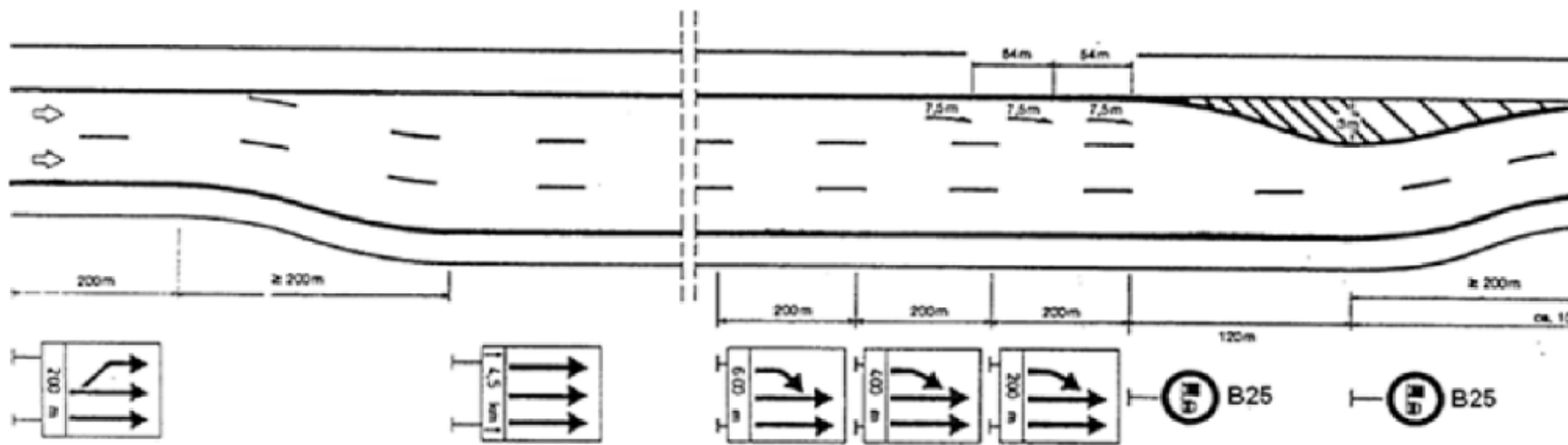
Фигура 12.2. Разположение и примерна сигнализация на допълнителна лента при нови автомагистралаи с разширяване на платното от страна на банкета
