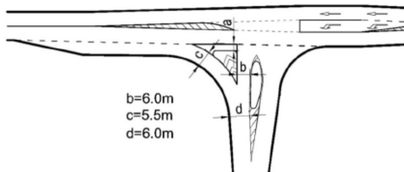
Фигура 57. Триъгълен остров
