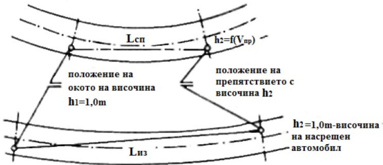
Фигура 9.3. Схематично положение на окото и на целевата точка (препятствието) при анализирането на разстоянията L_{сп} и L_{из} Таблица 9.1
