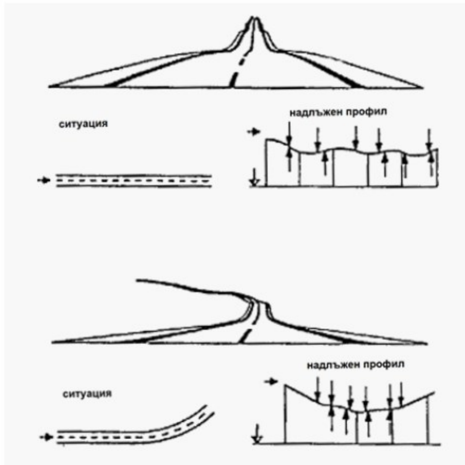
Фигура 23. Оптическо трептене
