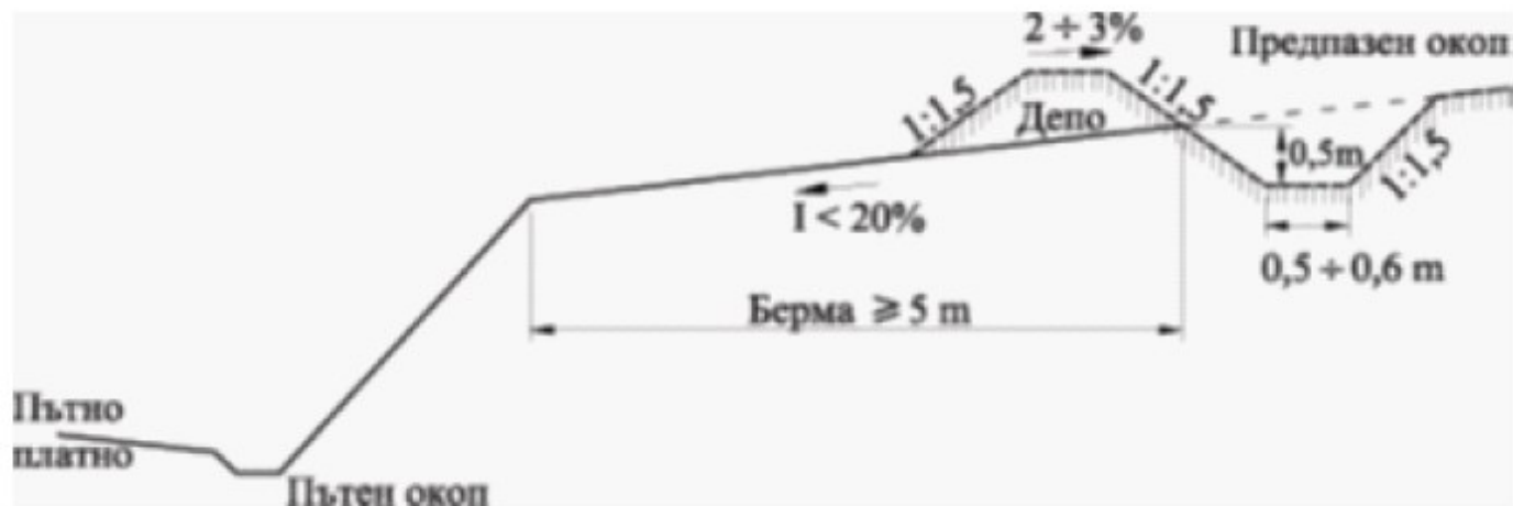
Фигура 111. Предпазен окоп
