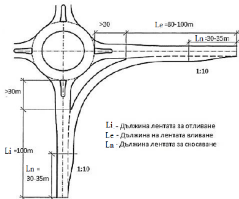
Фигура 65. Байпас на кръгово кръстовище
