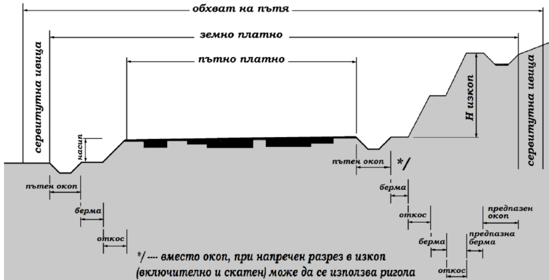
Фигура 29. Схематичен напречен профил
