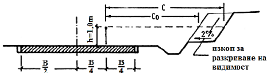
Фигура 10.1. Графична проверка за осигуряване на видимост в хоризонтална крива
