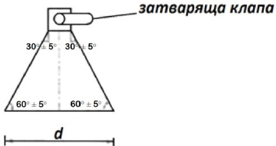
Фигура 18.2. Основна долна част на уред за определяне на обемната плътност чрез заместващ пясък
