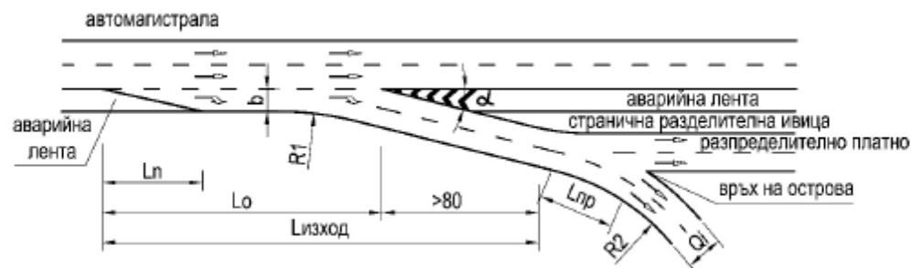
Фигура 93. Изход при разпределително платно (2) Дължината на участъка за отливане L_0 се определя съгласно таблица 32.
