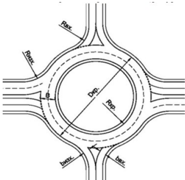
Фигура 50. Кръстовица от IV тип (кръгови кръстовица)
