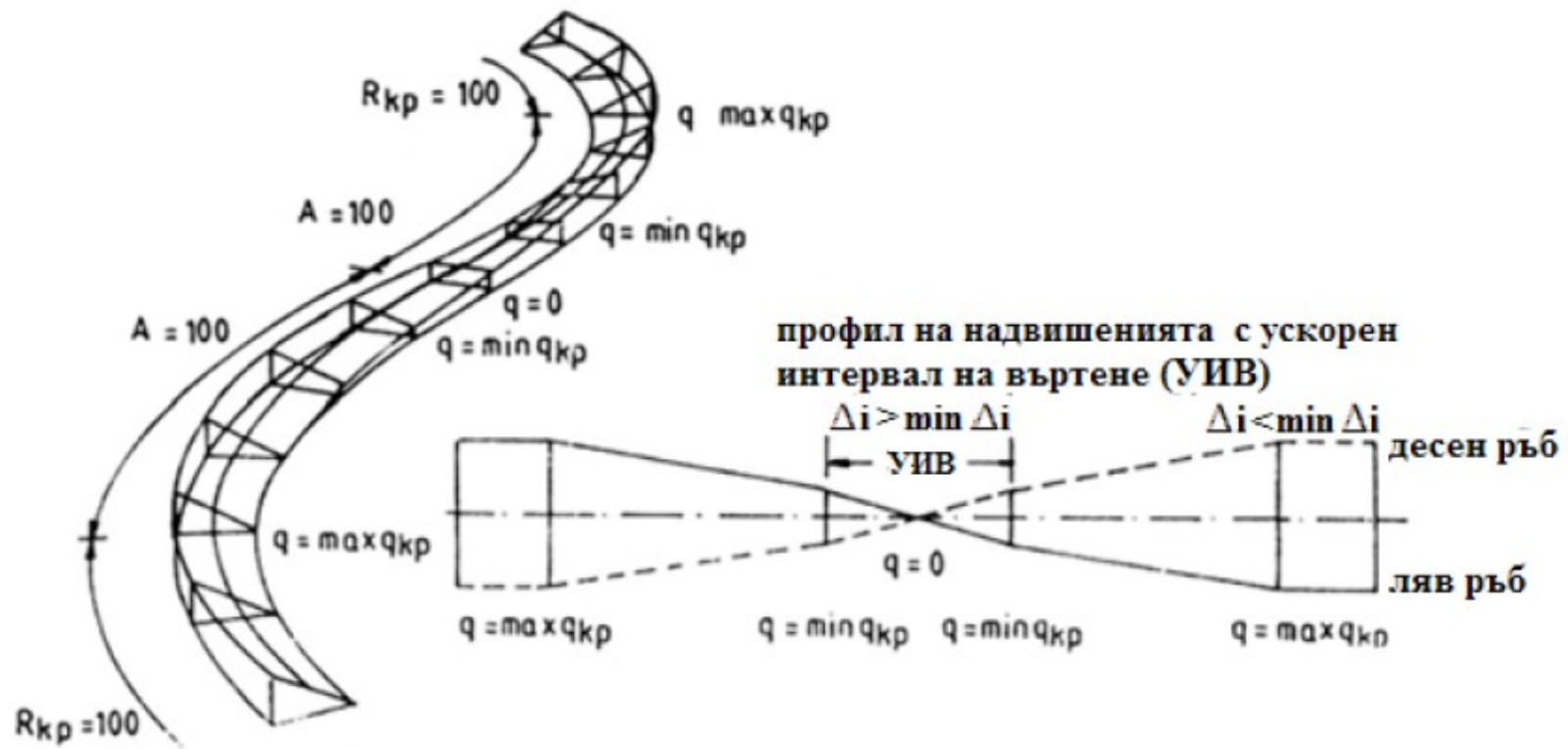
Фигура 8.2. Дълга отсечка на преоформяне
