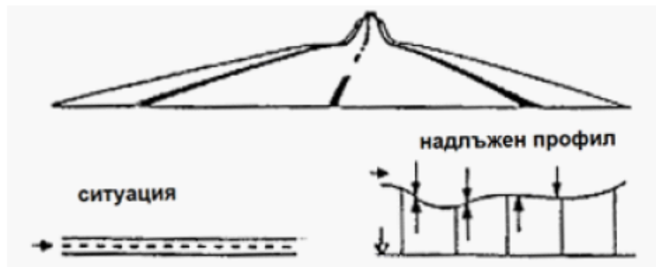
Фигура 22. Оптическо издуване
