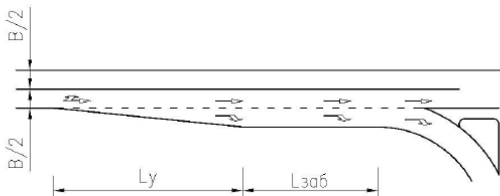
Фигура 52. Допълнителна лента ДД
